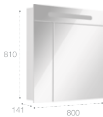
Общая ширина зеркального шкафчика 800 мм в открытом положении составит 1050 мм.
