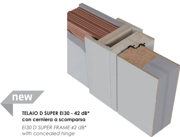
TELAIO EI30 con cerniera a scomparsa e/o a bandella EI30 FRAME with flap concealed hinge
