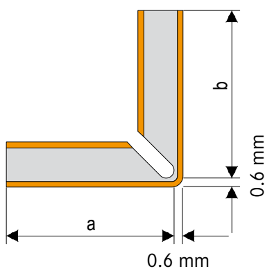
Fig. Exterior corner 90 °
