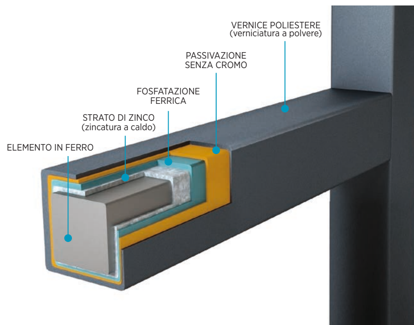
Sezione di un elemento protetto dal sistema DUPLEX .
