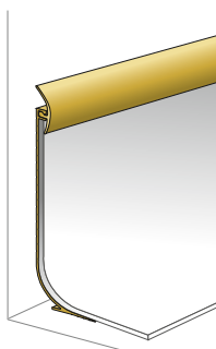
Sistema clip per curva di rimontatura completa
