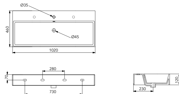
cod. ZELAVBW102 Lavabo Zenith bordo fino cm102 Zenith washbasin cm102 thin edge
