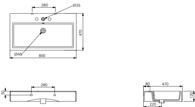
cod. QULAV80 Lavabo Quad cm80 Quad washbasin cm80
