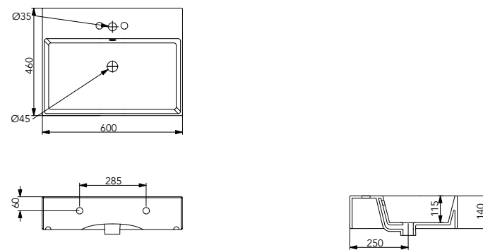
cod. ZELAVBW60 Lavabo Zenith bordo fino cm60 Zenith washbasin cm60 thin edge
