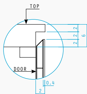
[IT] Particolare tecnico della giunzione tra top e anta.
