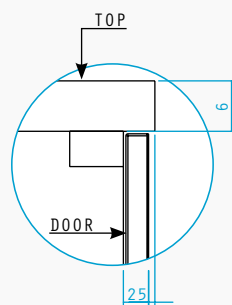
[IT] Particolare tecnico della giunzione tra top e anta.
