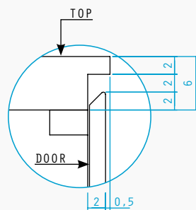
[IT] Particolare tecnico della giunzione tra top e ante.
