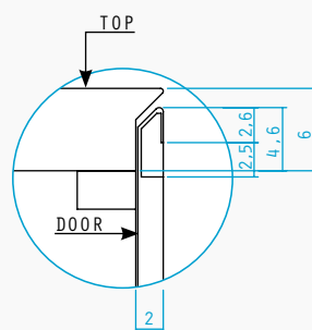
[IT] Particolare tecnico della giunzione tra top e anta.
