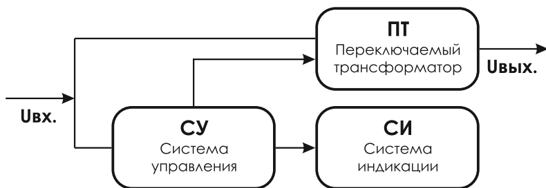
Структурная схема стабилизатора
